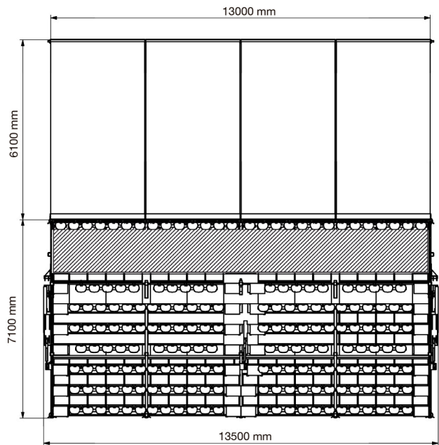
Vista Planta tribuna sin techo.
