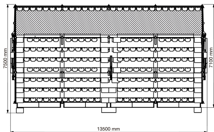
Vista Planta tribuna sin techo.
