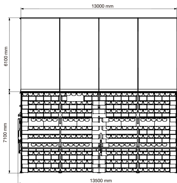
Vista Planta tribuna sin techo.
