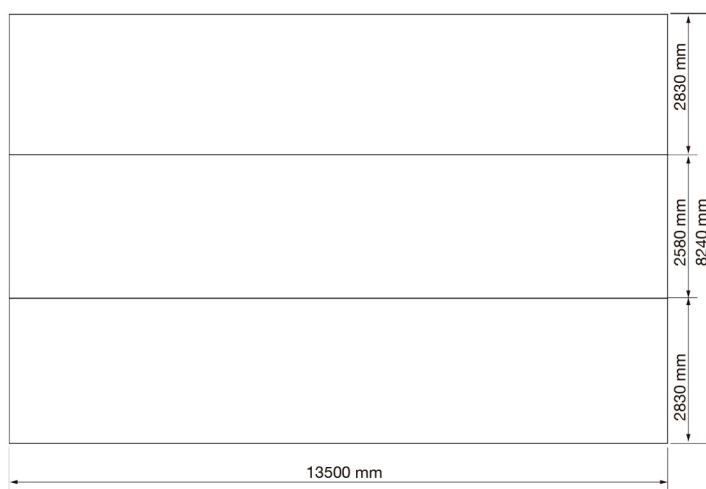
Vista Planta del techado tribuna.
